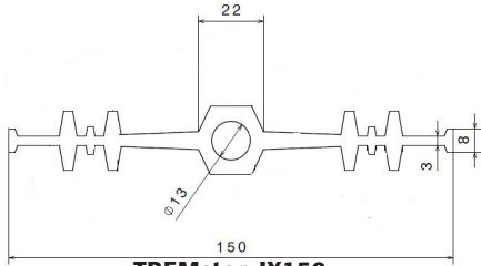
TREMstop IX150
