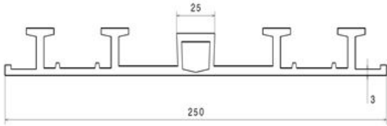
TREMstop EX250
