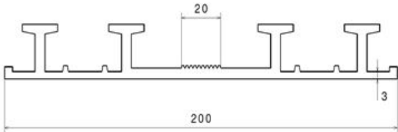
TREMstop EC200
