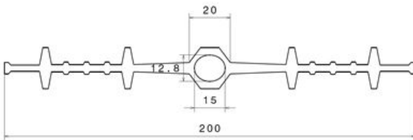
TREMstop IX200
